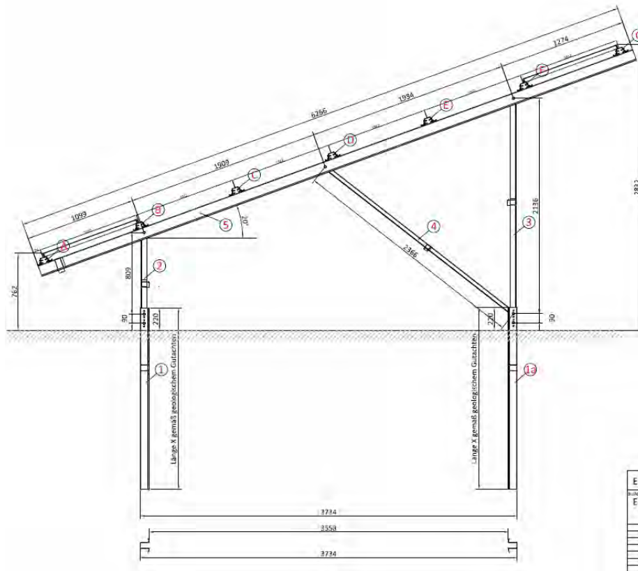
Abbildung 1.2 Darstellung Gestellstisch
